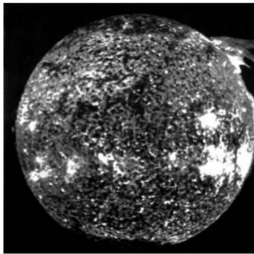
Sorprendente erupción solar. Fotografía tomada con luz ultravioleta desde la estación Skylab, 1973.
