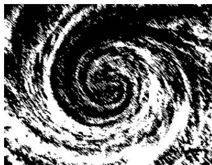
Galaxia típica en espiral, M-100.
